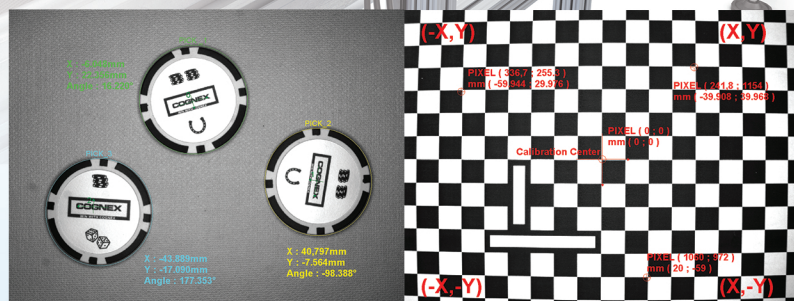
Esempio di presa con cordinarte XY e calibrazione guidata con scacchiera
